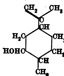
Carvomenthene.
